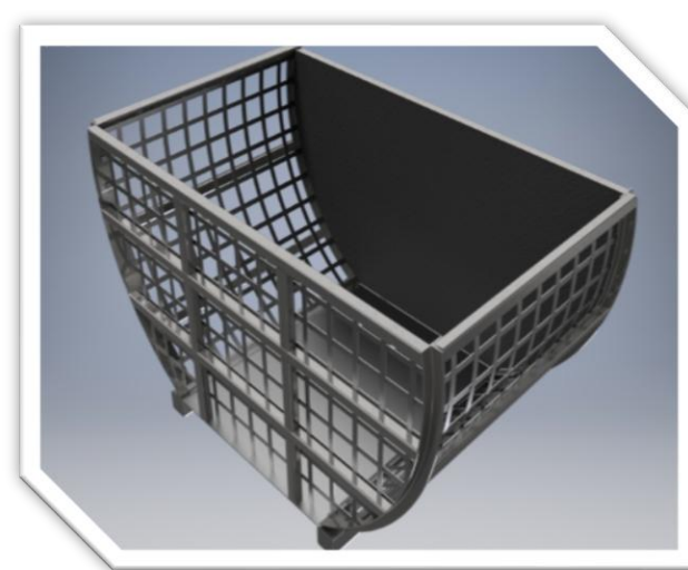
DISEÑO Y FABRICACION DE CANASTILLA PARA PIÑAS DE AGAVE
